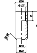
Līdzda "H" (M1:2)
